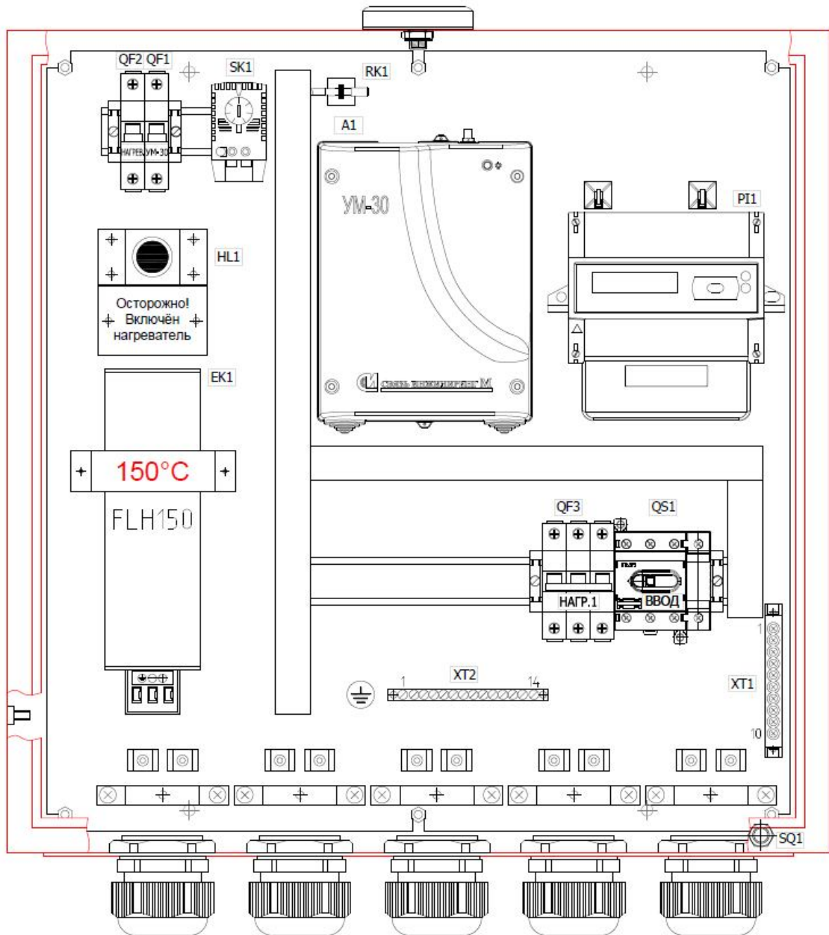
Рисунок 2 – Общий вид размещения оборудования в щите
