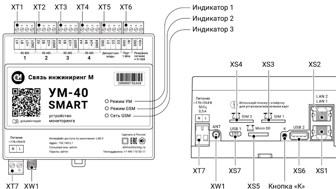
Рисунок 3 – Расположение разъёмных соединителей, индикаторов и кнопок
