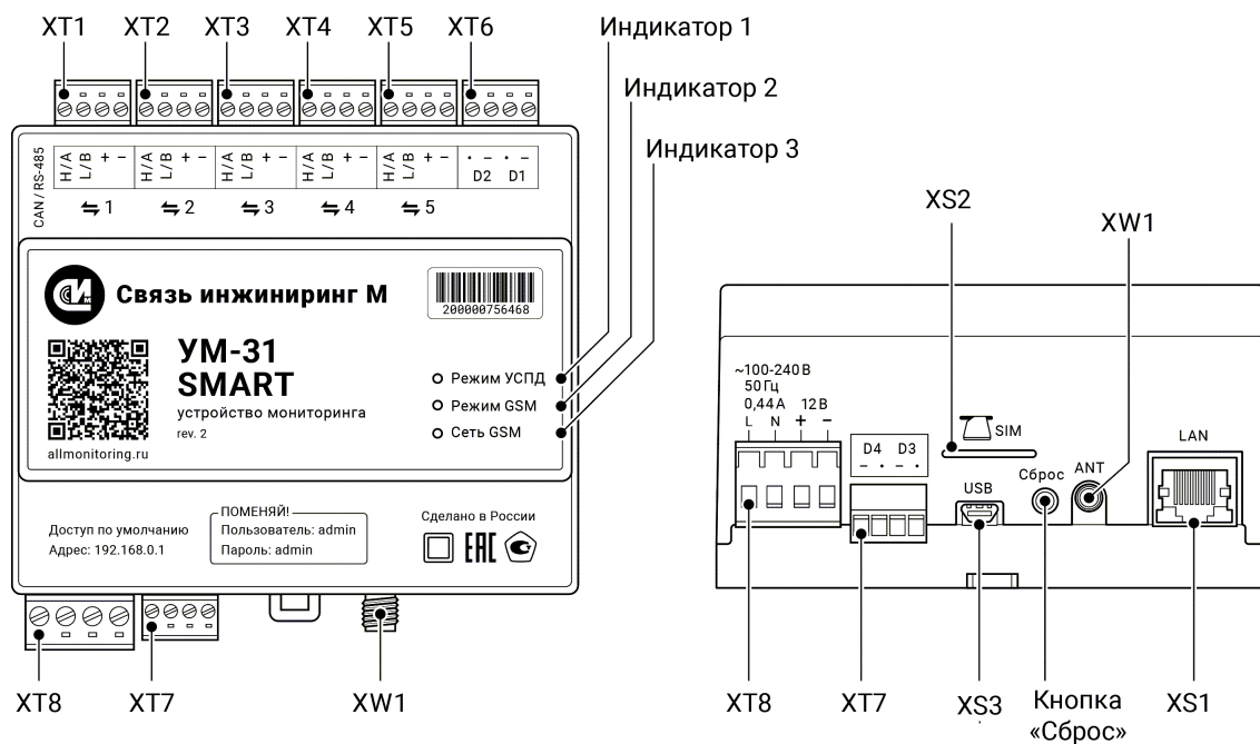
Рисунок 2. Расположение клеммников, индикаторов и кнопки «Сброс»
