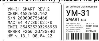
Рисунок 6. Формат наклейки
