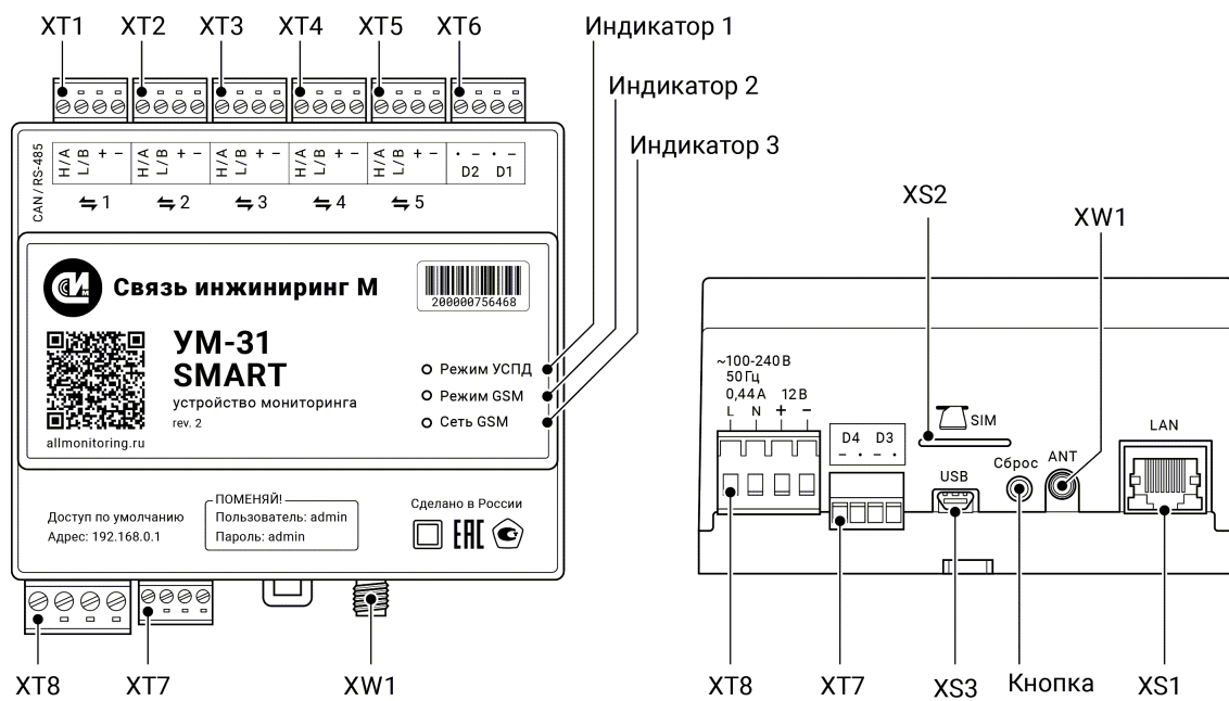
Рисунок 2. Расположение клеммников, индикаторов и кнопки «Сброс»
