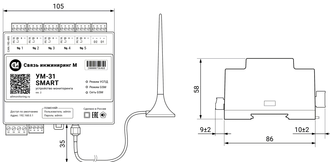
Рисунок 1. Габаритные размеры устройства
