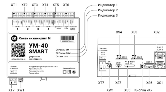
Рисунок 2. Расположение клеммников, индикаторов и кнопок
