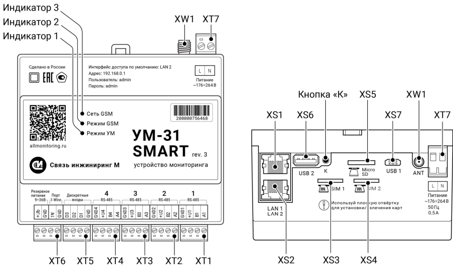
Рисунок 2. Расположение клеммников, индикаторов и кнопок
