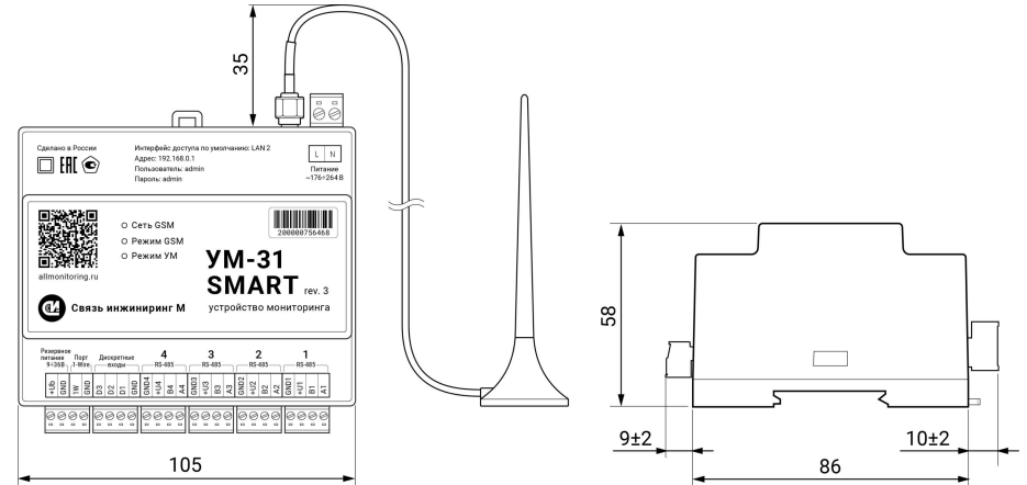
Рисунок 1. Габаритные размеры устройства
