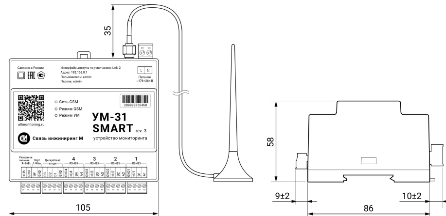
Рисунок 1. Габаритные размеры устройства
