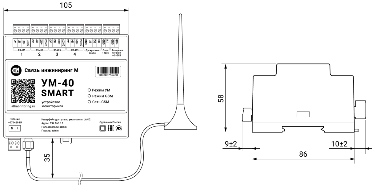
Рисунок 1. Габаритные размеры устройства
