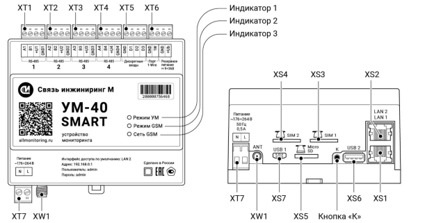
Рисунок 2. Расположение клеммников, индикаторов и кнопок
