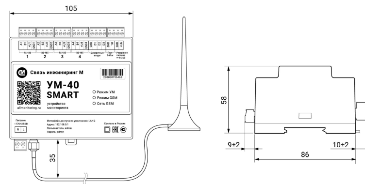
Рисунок 1. Габаритные размеры устройства
