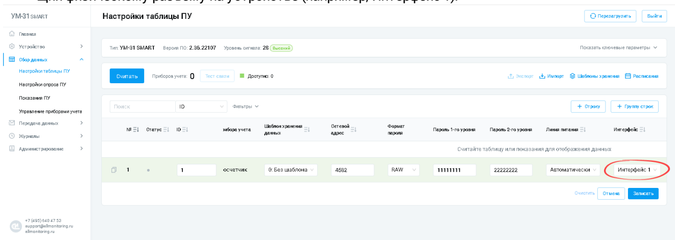
Рисунок 4. Интерфейс 1
