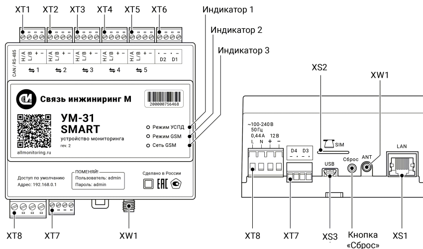
Рисунок 2. Расположение клеммников, индикаторов и кнопки «Сброс»
