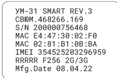
Рисунок 3. Формат наклейки
