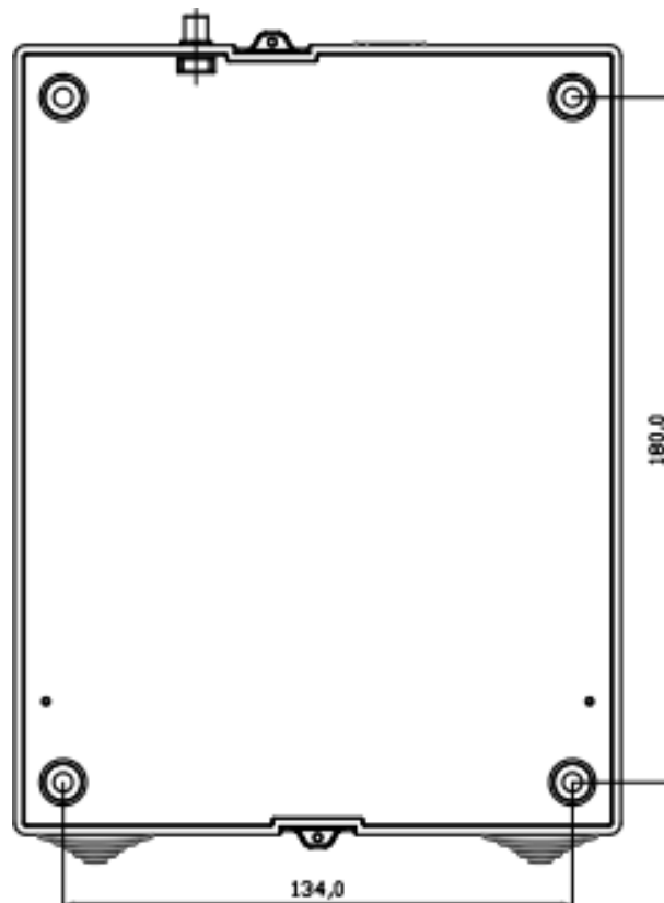
Рисунок 5. Установочные размеры
