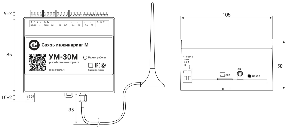
Рисунок 1. Габаритные размеры устройства
