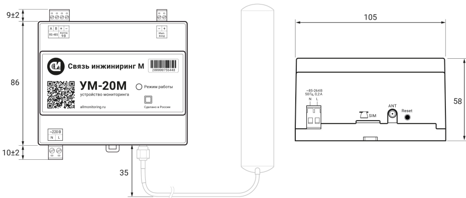
Рисунок 1. Габаритные размеры устройства
