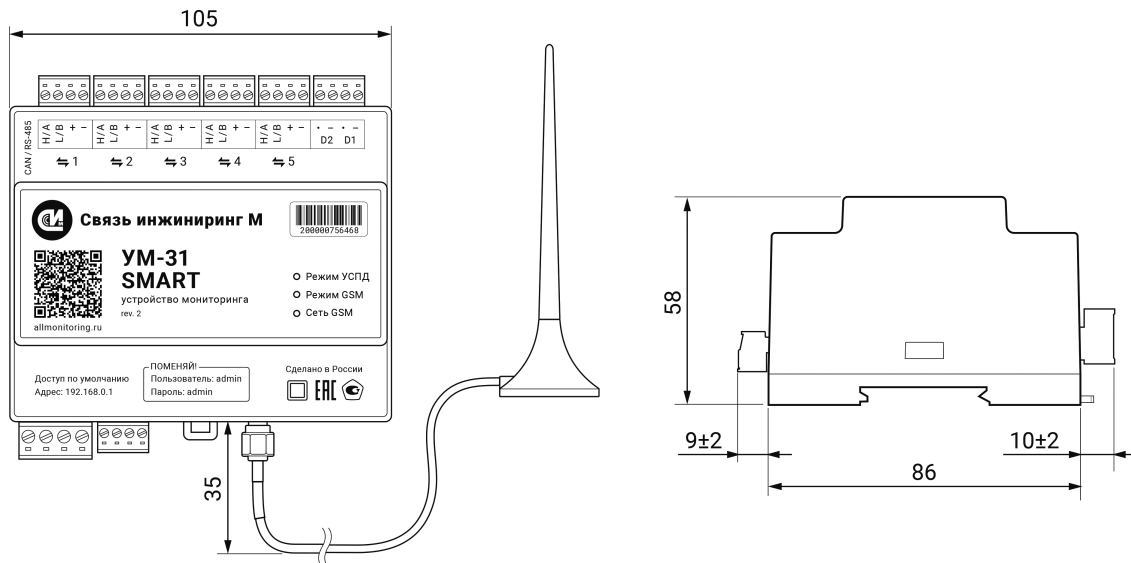
Рисунок 1. Габаритные размеры устройства
