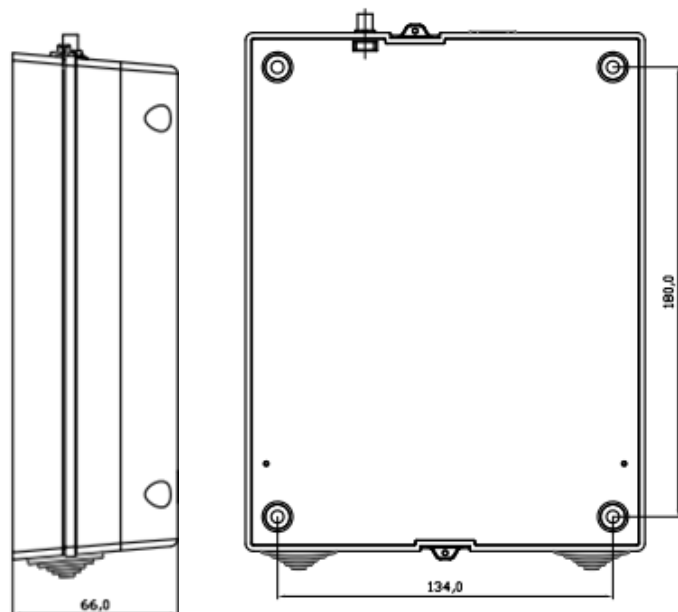
Рисунок 5. Установочные размеры
