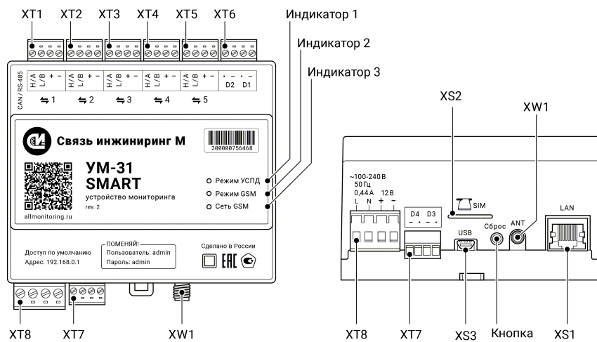
Рисунок 2. Расположение клеммников, индикаторов и кнопки «Сброс»
