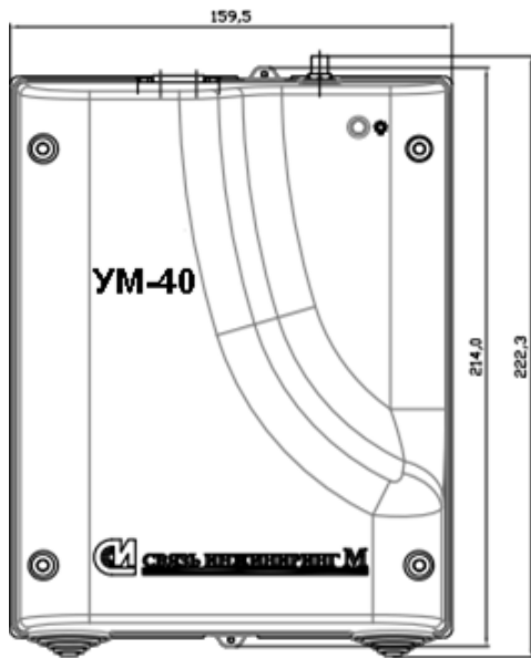
Рисунок 4. Габаритные размеры
