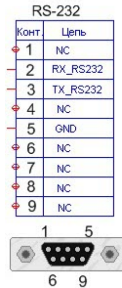
Рисунок 1. Описание разъёма RS-232
